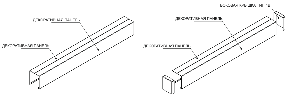
УСТАНОВКА НА ПРОЕМ
