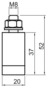
фиксатор троса фасадный
